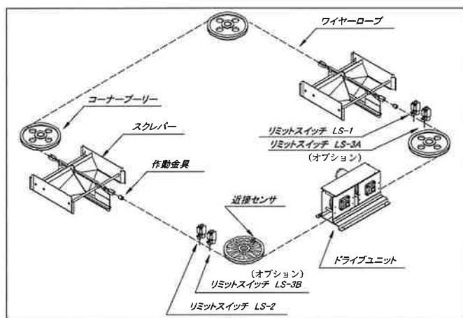
【ピットクリーナー複列型 VW】
