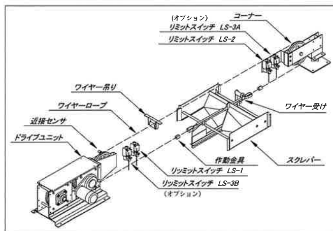
【ピットクリーナー単列型 VS】
